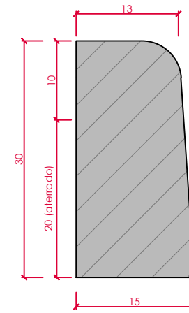
DETALHAMENTO MEIO-FIO SEM ESCALA
