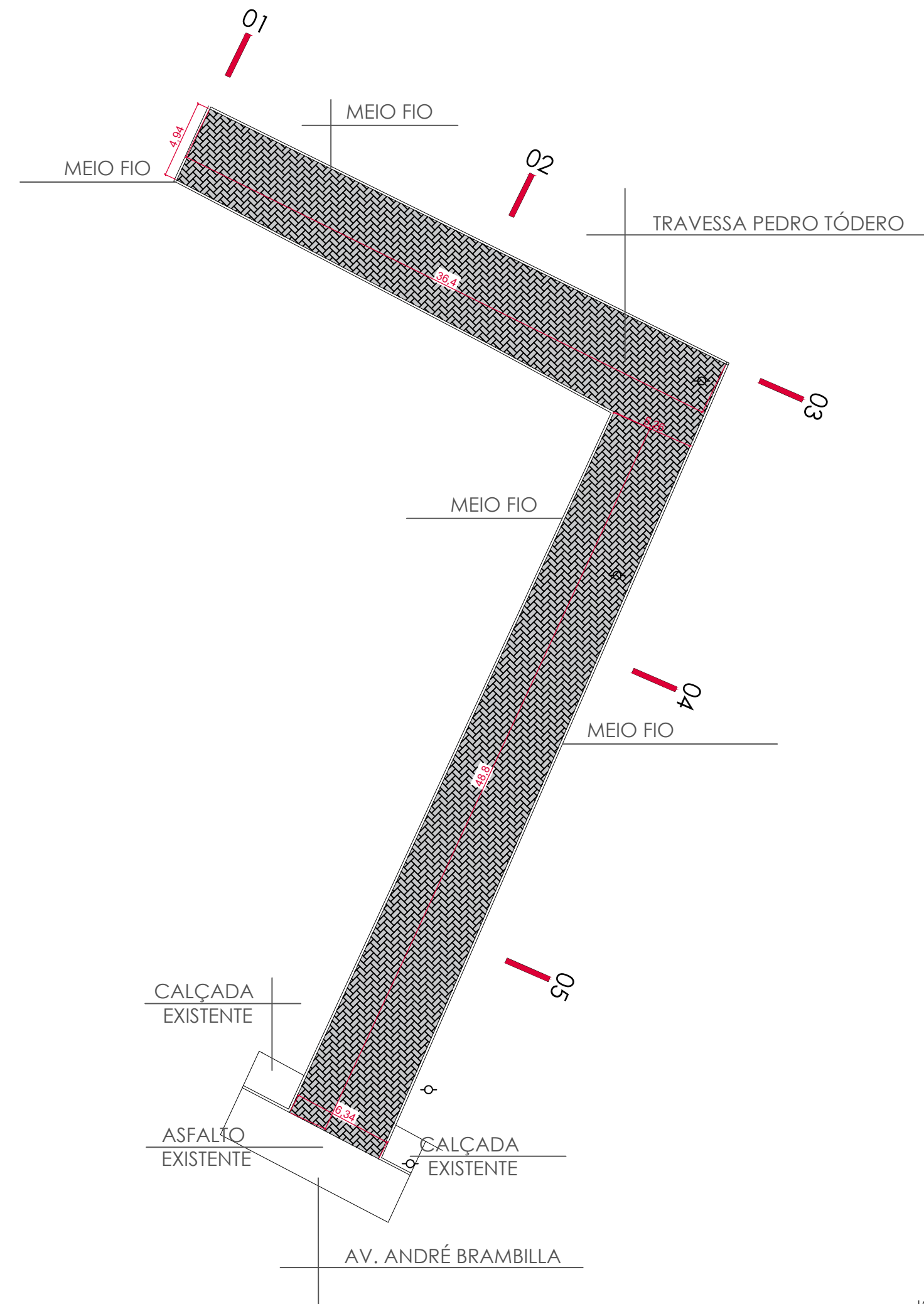
DETALHAMENTO 05 | PAVIMENTO SEM ESCALA
