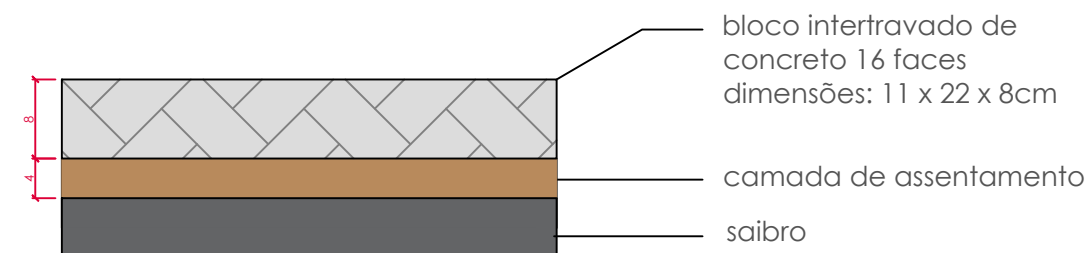
DETALHAMENTO 05 | PAVIMENTO SEM ESCALA
